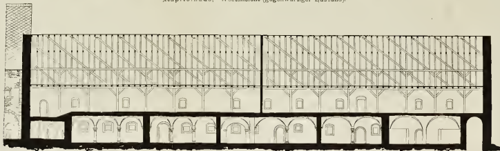
Kapitelsaal, Längsschnitt (Zustand vor 1882)
